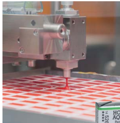
Befüllung der Näpfchen Filling of watercolour pans
